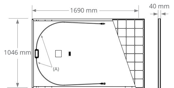
PROFILE CADRE
